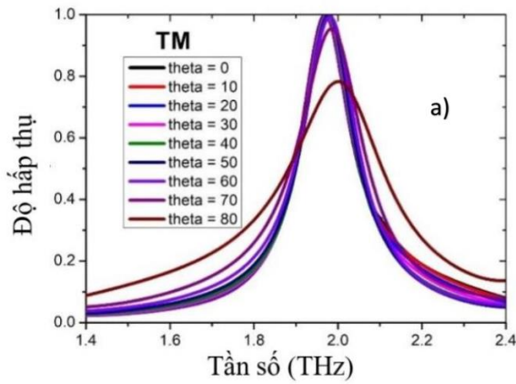
Độ hấp thụ của siêu vật liệu MMA tích hợp Graphene với các góc khác nhau của sóng tới. a) Phân cực từ TM; b) Phân cực điện TE.
